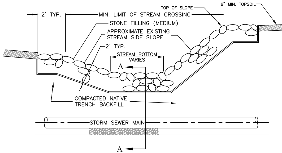
LONGITUDINAL SECTION
