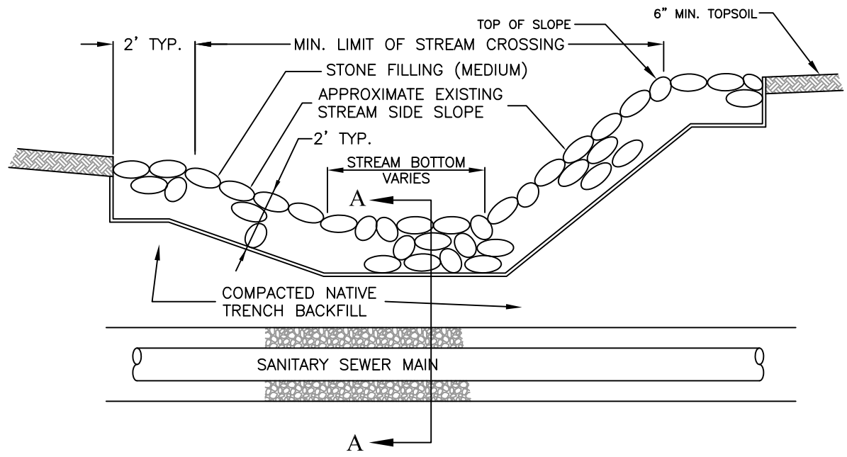
LONGITUDINAL SECTION
